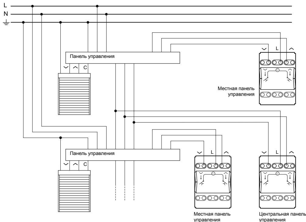
3-10 АХ, кнопочный выключатель Н.О. контакт (1-2), ОСТАНОВКА (1+2) для автоматизации – S5xx227
