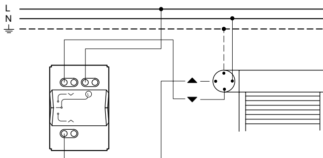
1-6 АХ, переключатель, 3 клавиши /3 положения – S5x
