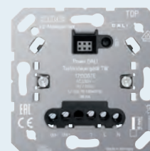
Кнопочный контроллер DALI с источником питания TW
